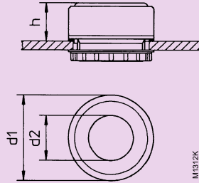
Indicating lamp bezel
