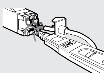
Wiring using the impact tool (110) แบบใช้อุปกรณ์เข้าสาย
