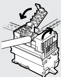
Wiring without tools (Toolless) แบบล็อกอัตโนมัติ
